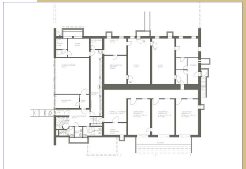
Plan des Untergeschosses.
